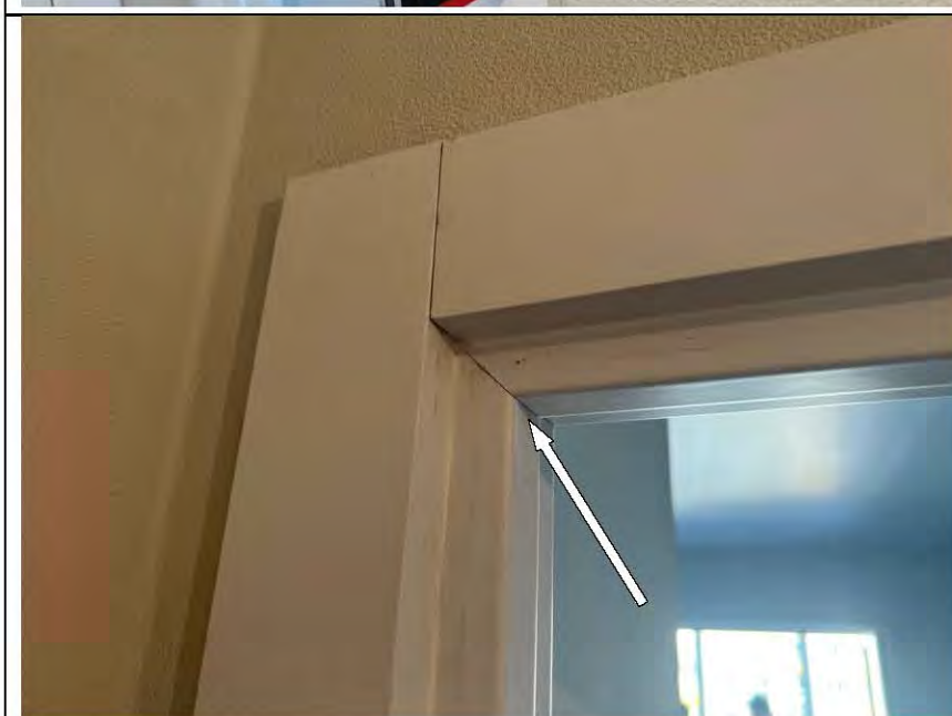
Фото №57. Элементы дверного блока в кухне соединены не надежно (коробка).
