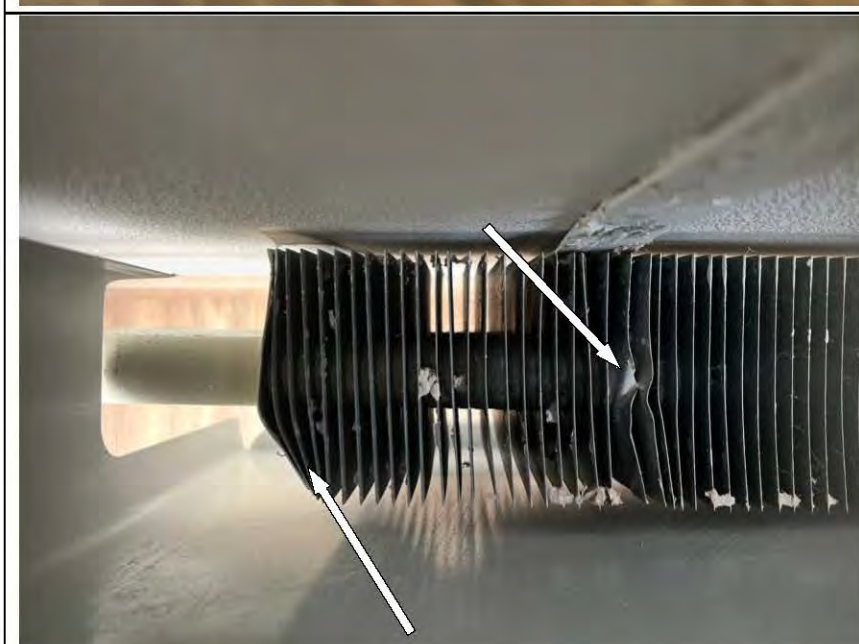
Фото №68. Замятие и загрязнение сот радиатора в спальне.
