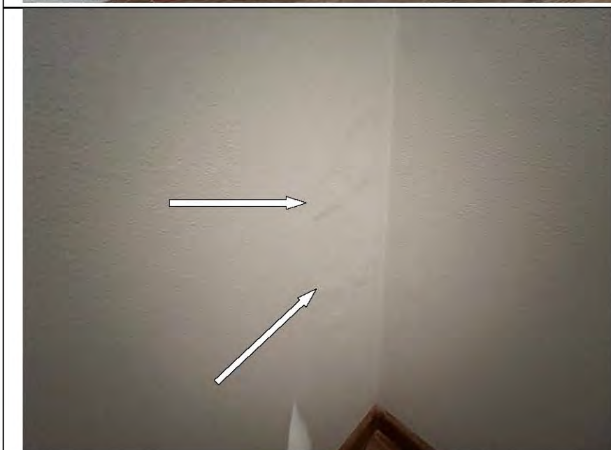
Фото №23. Отслоение обойного полотна в гардеробной.
