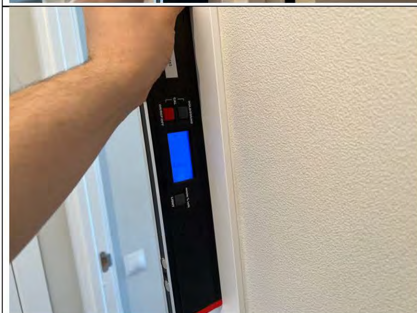
Фото №56. Отклонение наличников дверного блока в кухне на 3 мм от вертикальной плоскости.
