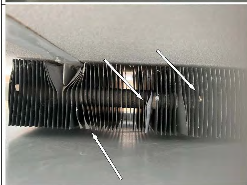
Фото №69. Замятие и загрязнение сот радиатора в лоджии.
