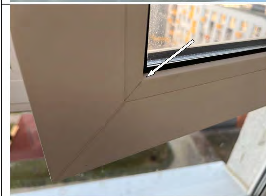
Фото №45. Зазоры в стыках профиля ПВХ оконного блока в лоджии.
