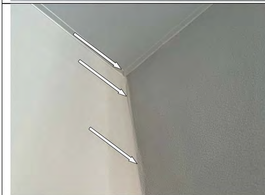
Фото №21. Отслоение обойного полотна в кухне. Соединение декоративного молдинга натяжного потолка в кухне выполнено некорректно.
