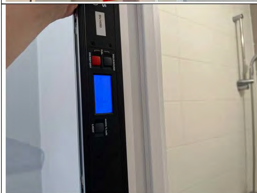
Фото №65. Отклонение коробки дверного блока в ванной комнате на 3 мм.
