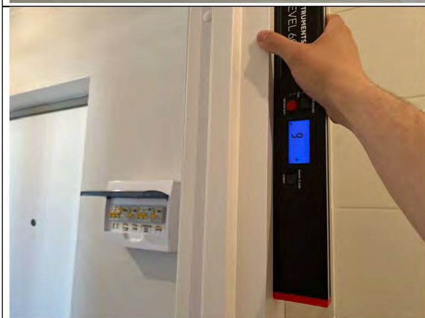
Фото №53. Отклонение наличников дверного блока в ванной комнате на 6 мм от вертикальной плоскости.
