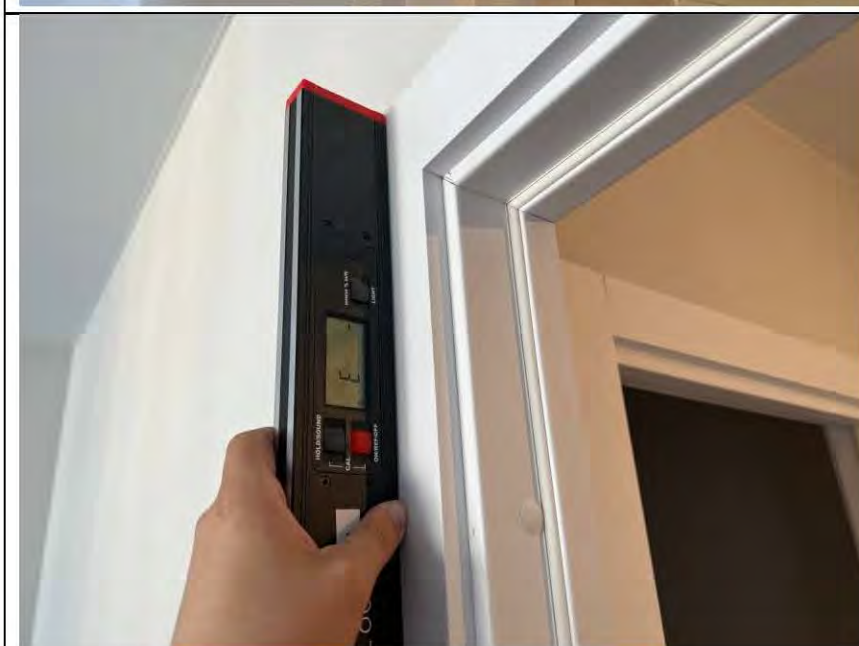
Фото №54. Отклонение наличников дверного блока в спальне на 3 мм от вертикальной плоскости.
