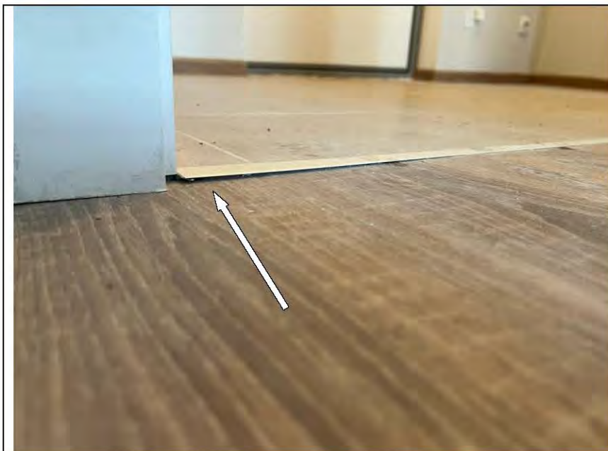
Фото №67. Щель между металлическим порогом и ламинатом в спальне.
