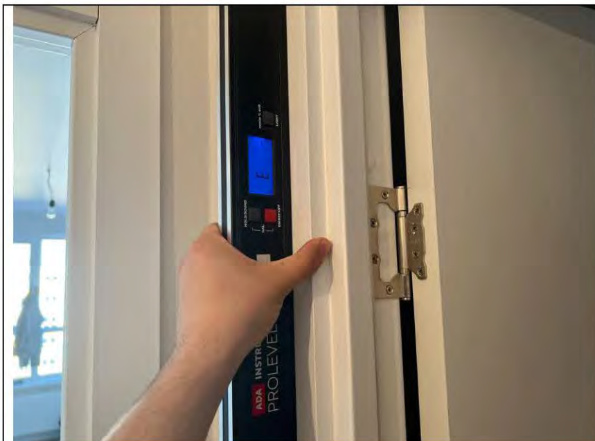
Фото №55. Отклонение наличников дверного блока в гардеробной на 3 мм от вертикальной плоскости.
